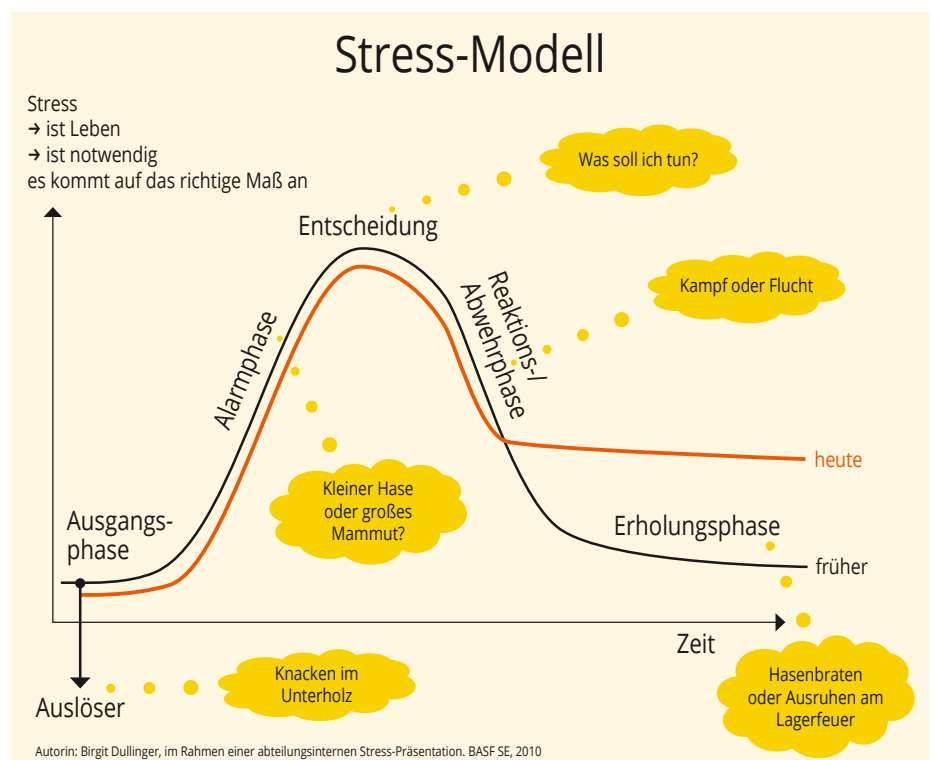
Abbildung 1: Ein Stress-Modell
